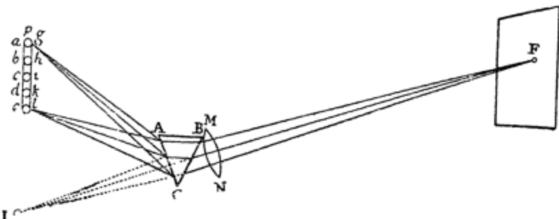
Рис. 16. Схема спектральной установки Ньютона.
