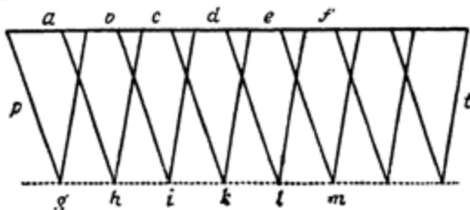
Рис. 17. Схема спектра, образуемого при треугольной щели.
