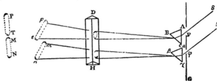
Рис. 18. Схема опыта Ньютона со скрещенными призмами.
