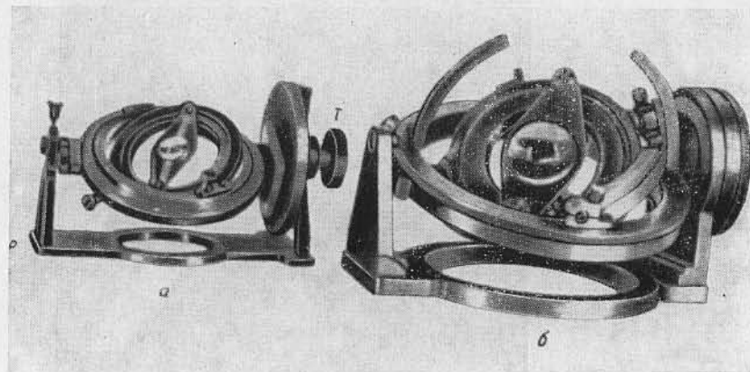
Федоровский столик: а) ранняя конструкция, б) современная.
