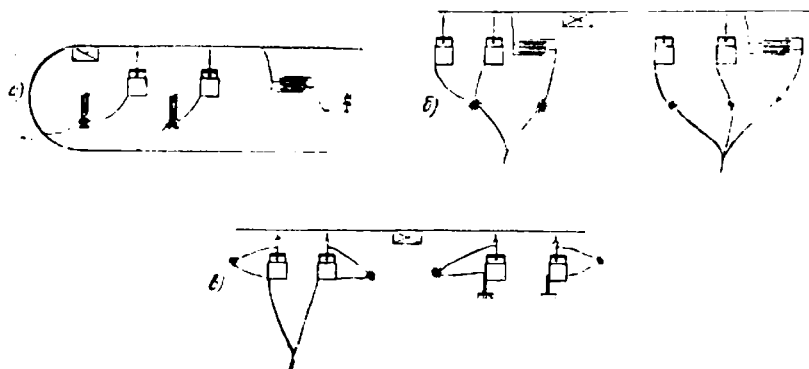
Черт. 7. Способ «дробления» электрического света с помощью конденсатора: а) включение источников света без посредства земли; б) за один полюс взята земля и источники света включены или между наружной обкладкой лейденской банки и землёю или параллельно лейденской банке; в) то же, причём в конденсаторе должно, по мнению Шлөблочкова, дополнительно аккумулироваться атмосферное электричество (наружная обкладка лейденских банок соединена с металлической гребёнкой для облегчения выхода электричества в воздух).
