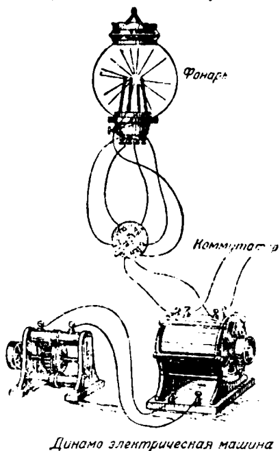
Черт. 5. Общая схема электрического освещения Яблочкова.
