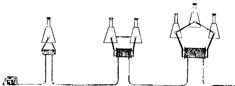
Черт. 6. Трансформаторы Яблочкова для питания нескольких источников света, независимо один от другого.
