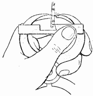
Фиг. 306. Разрезной баланс с нарушением плоскостности.
