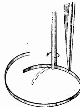
Фиг. 159. Способ обрыва внутреннего витка спирали.
