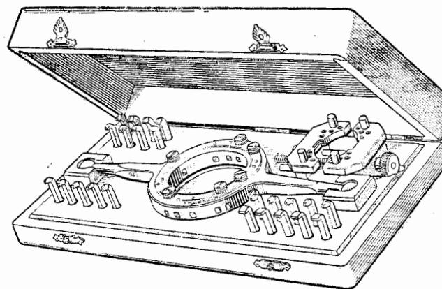
Фиг. 435. Швейцарский набор универсальных инструментов «Vergeon» для открывания корпусов.
