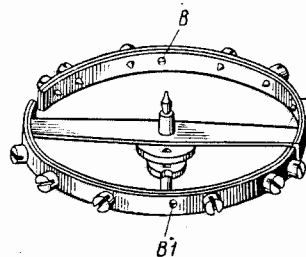
Фиг. 144. Температурная регулировка, выполняемая для того, чтобы часы спешили при высокой температуре. B, BI — отверстия для компенсационных винтов.
