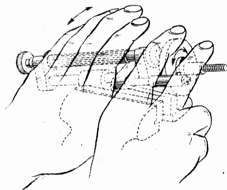
Фиг. 358. Приспособление для обработки головок винтов вручную.
