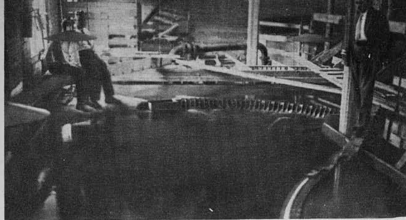
Модель узла Днепростроя в Гидравлической лаборатории ЦАГИ.
