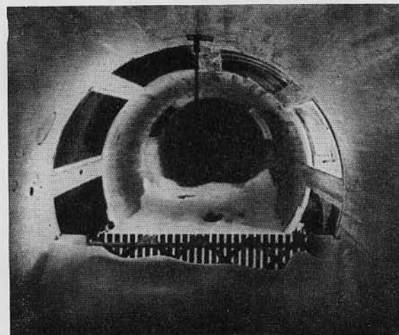
Изучение снежных за- носов в аэродинами- ческой трубе.
