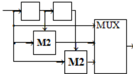
Рис. 3.7 – Схема кодера систематического сверточного кода для k/n = 1/3
