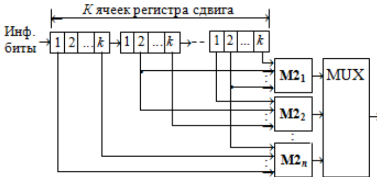
Рис. 3.6 – Общая схема кодера сверточного кода со степенью кодирования k/n
