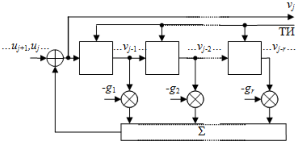
Рис. 2.11 – Рекурсивный цифровой фильтр
