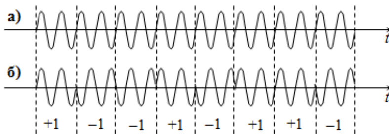
Рис. 6.8 – Преобразование информационного импульса в сигнал с внутриимпульсной ФМ:
