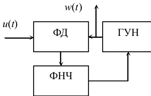
Рис. 5.5 – Генератор опорного колебания с петлей ФАПЧ
