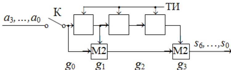
Рис. 3.3 – Схема кодера несистематического (7, 4) -кода на основе производящего полинома
