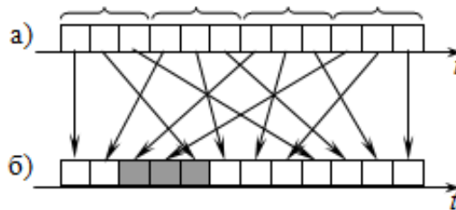
Рис. 3.8 – Схема, иллюстрирующая табличный способ перемежения по времени ( n = 3, m = 4 ):
