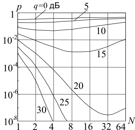
Рис. 5.10 – Зависимость битовой вероятности ошибки при различении двух равновероятных ортогональных сигналов от кратности разнесения при различных значениях отношения сигнал/шум
