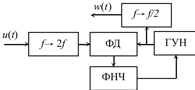
Рис. 5.6 – Генератор опорного колебания с петлей ФАПЧ на удвоенной несущей частоте
