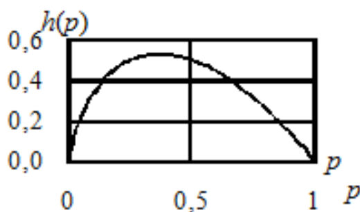
Рис. 4.1 – Вспомогательная функция h(p) = -p \log_2 p
