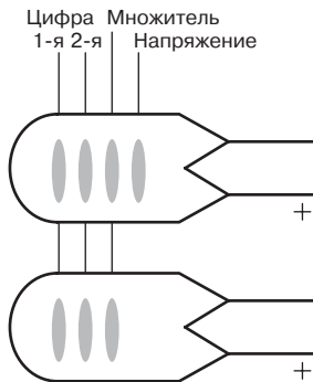
Рис. ПЗ.6. Цветовая маркировка танталовых конденсаторов
