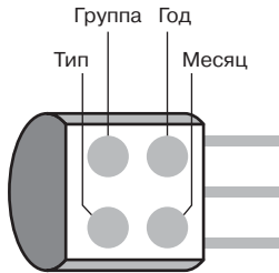
Рис. ПЗ.11. Маркировка транзисторов четырьмя цветными точками
