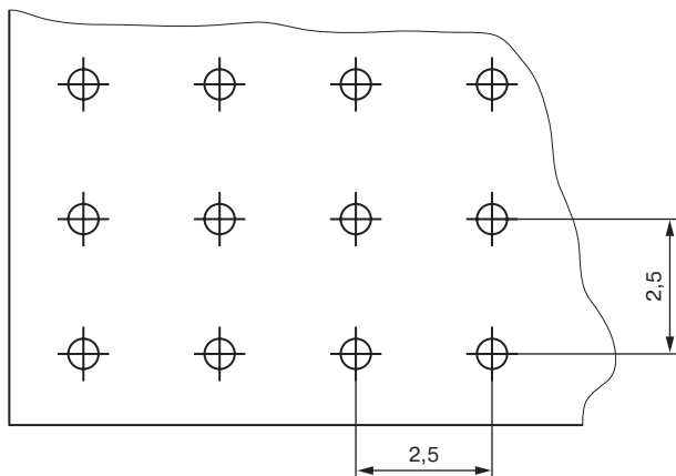
Рис. 3.1. Пластина-шаблон
