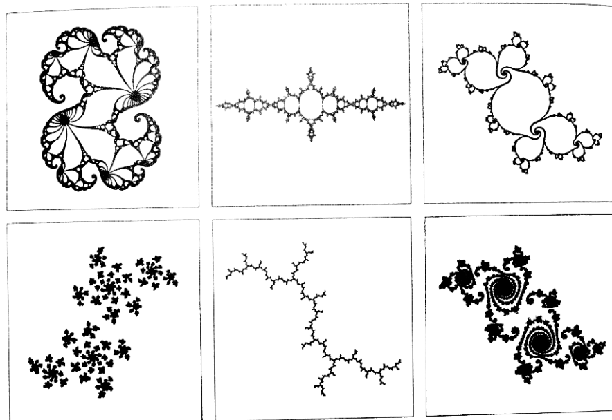
Рис. 6. Примеры множеств Жюлиа (Пайтген, Рихтер, 1993)
