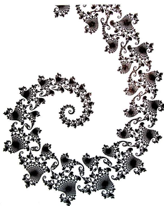
Рис. 9. Фрагмент множества Мандельброта , полученный с увеличением разрешающей способности компьютера (Пайтген, Рихтер, 1993)
